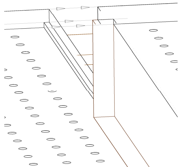
Detalle de ensamblaje / Assembly detail
